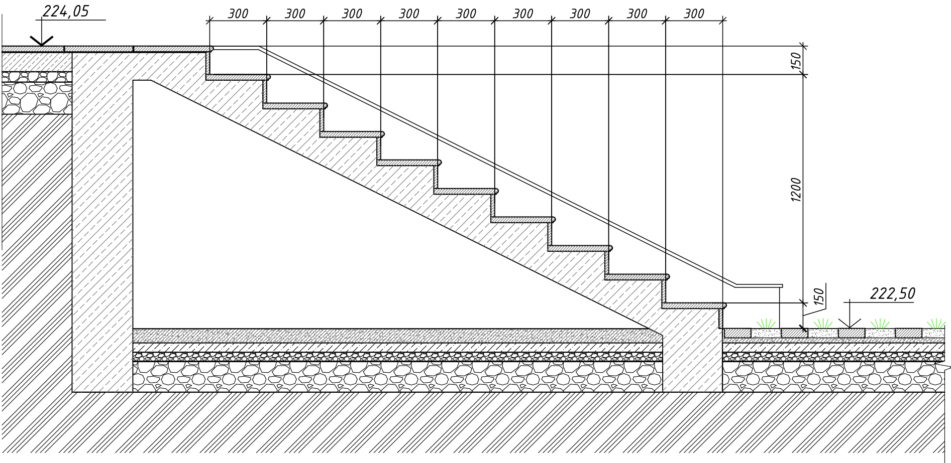
Лестница 1
