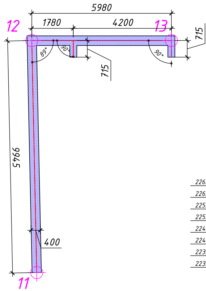
Подпорная стена 1
