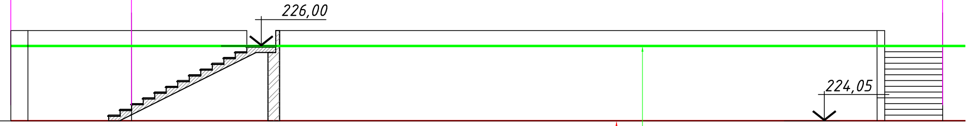
Подпорная стена 3
