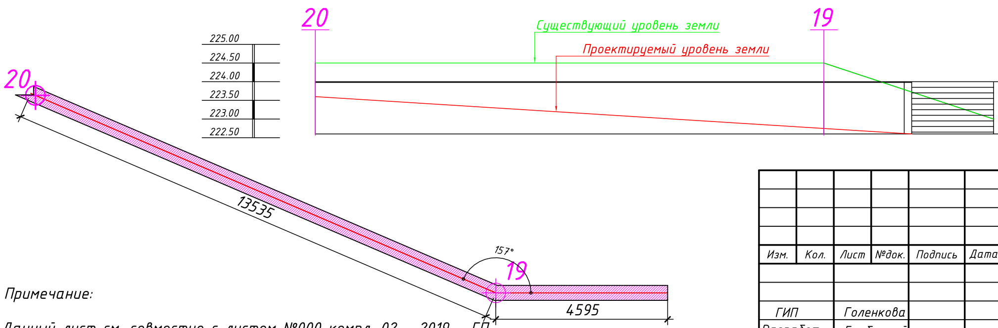
Подпорная стена 4
